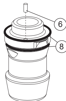
MTS Ausgleichzapfen / A MTS compensation spigot / A Tige de compensation / A MTS
