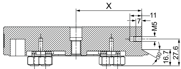
Schnitt A - A
